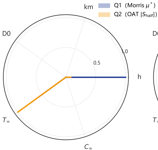
(a) 输出 T(R)
